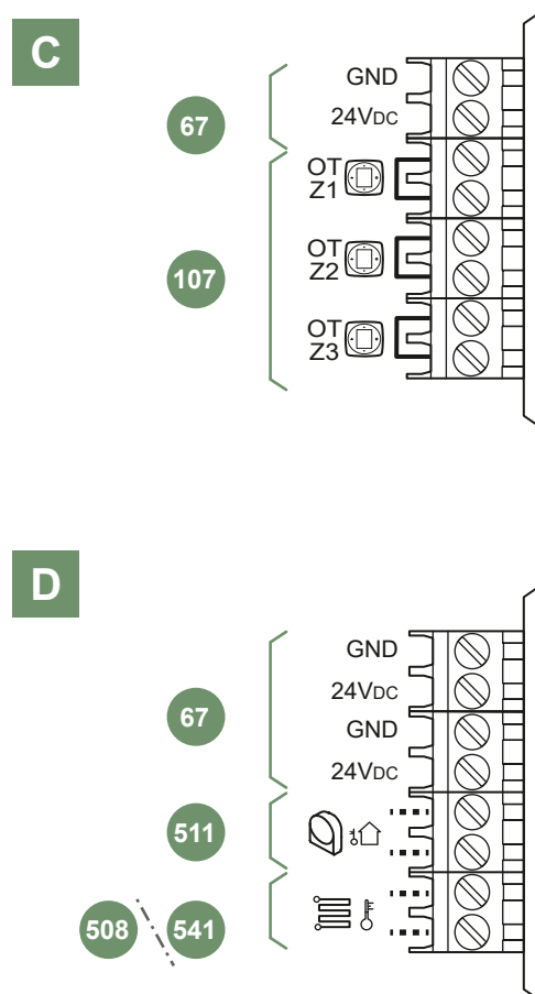
fig. 13 - Aansluiting op de klemmenstrook
