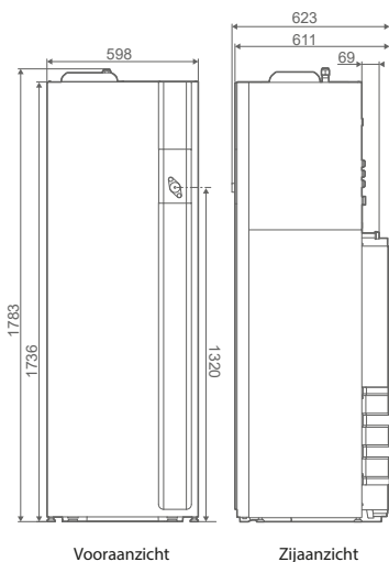
Vooraanzicht
