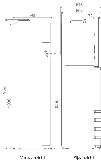
Vooraanzicht
