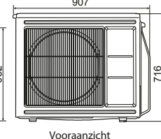
Vooraanzicht
