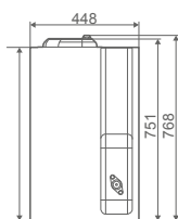
Vooraanzicht
